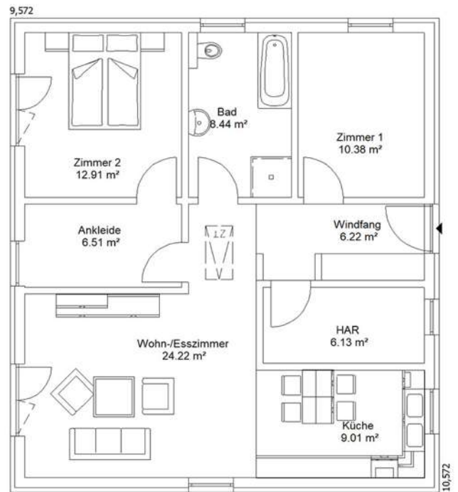
Erdgeschoss 83,82 m 2
